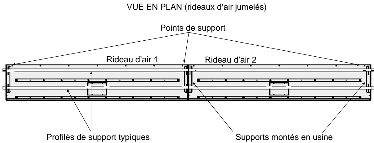
Diagramme 4: profile de support (rideaux d'air multiples)
