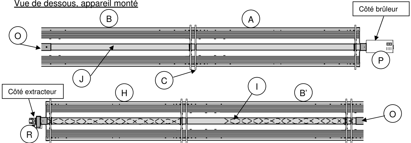
Vue de dessous, appareil monté
